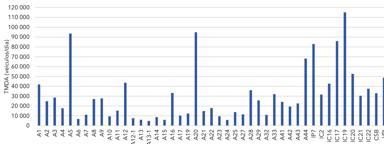
Gráfico 5. Tráfego Médio Diário (TMDA) em 2023, por autoestrada
