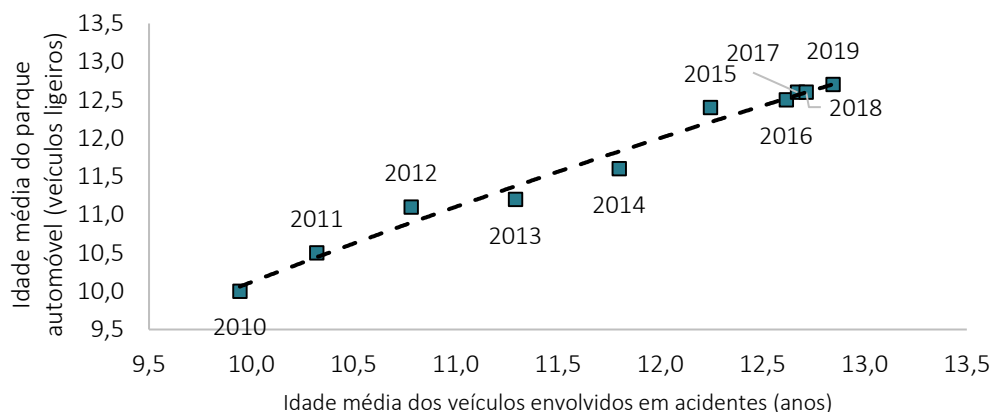
Figura 64: Relação entre a idade média do parque automóvel e a idade média dos veículos envolvidos em acidentes
