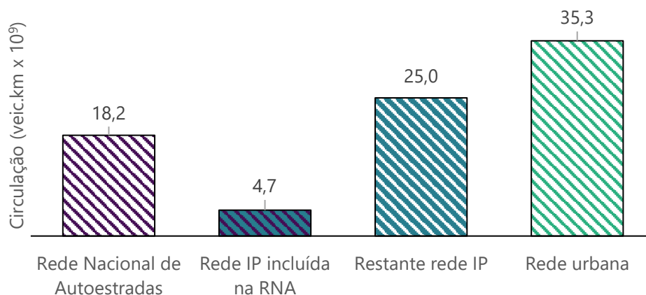
Figura 50: Circulação anual (veic.km x 10 9 ) em cada tipo de rede
