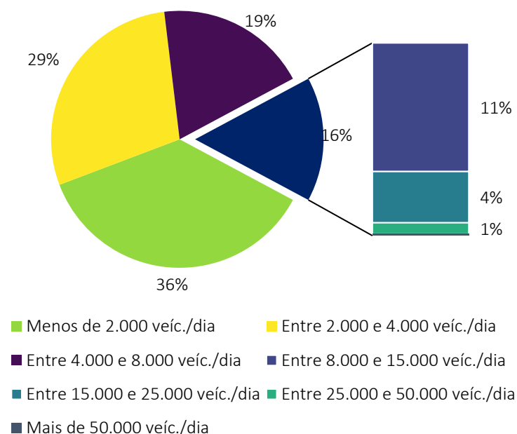
Figura 49: Níveis de tráfego médio diário anual (TMDA) na restante rede IP (sem RNA)
